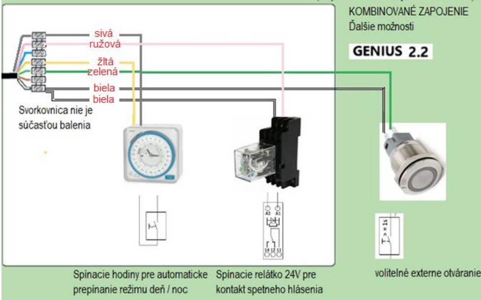
EI. rozbočovacia krabica s DIN lištou (nie je súčasťou dodavky. Zabezpečí stavba)
